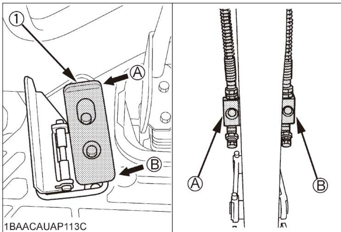
(1) AUX1 (サービスポート) ペダル
